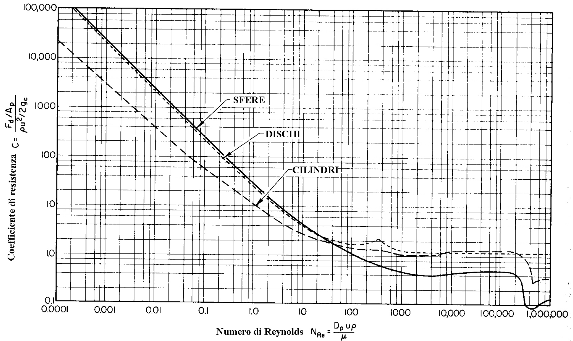
Coefficiente di resistenza aerodinamico per sfere, dischi e cilindri investiti ortogonalmente da un flusso d'aria.
