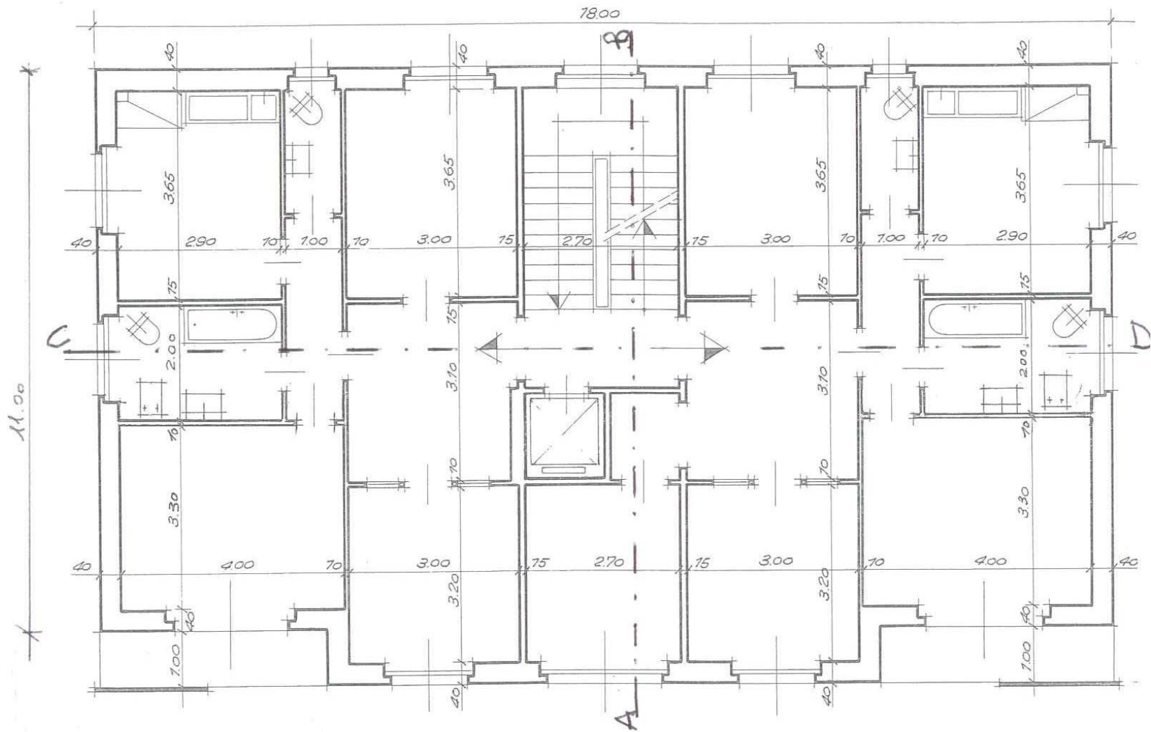
Fig. 71 - Esempio di una pianta nella quale non risultano indicati i pilastri.
